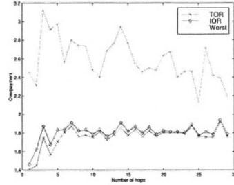
(d) the affect of hops on IOR, TOR and WOR
